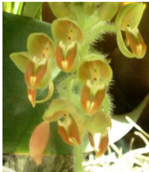
Pontieva sp.
